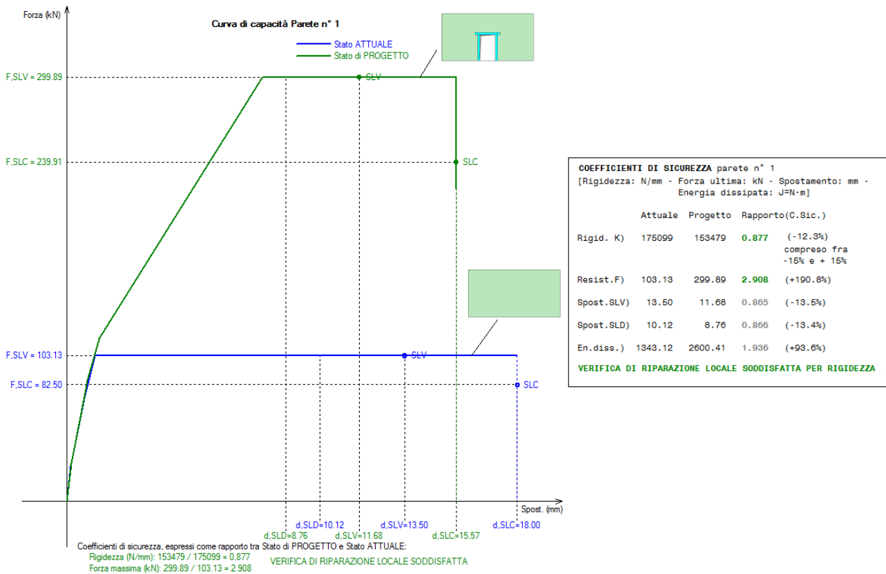
Fig. 5. Risultati dell'analisi locale della parete su modello 2D
