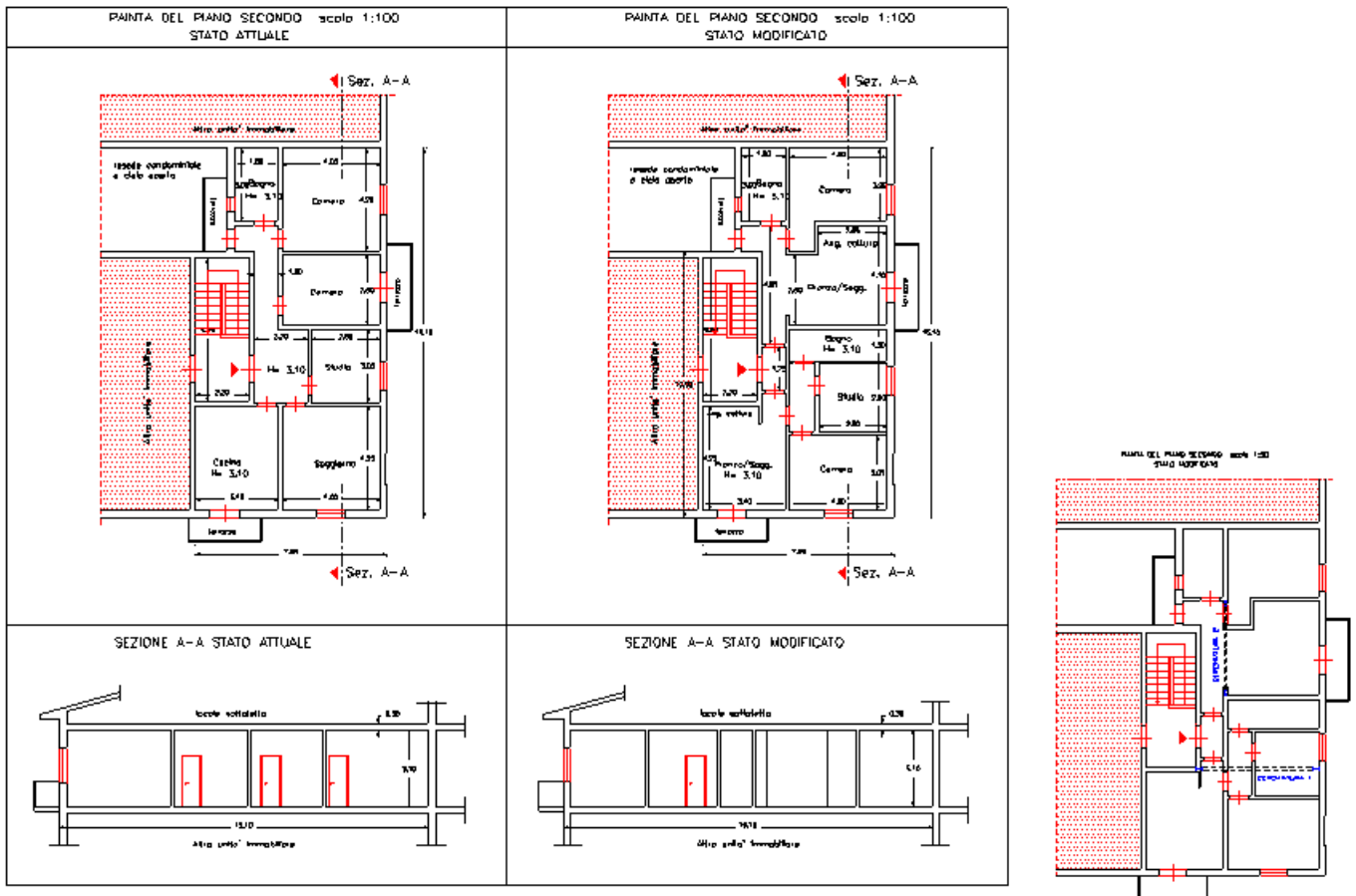
Fig. C.2.1. Pianta e Sezioni Stato Attuale e Stato Modificato
