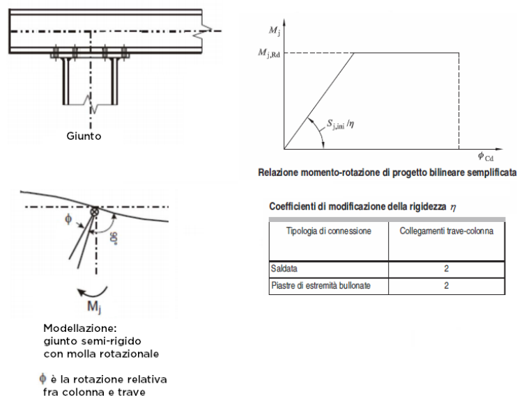
Fig. B.5.11. Giunto: comportamento bilineare elastico-perfettamente plastico
