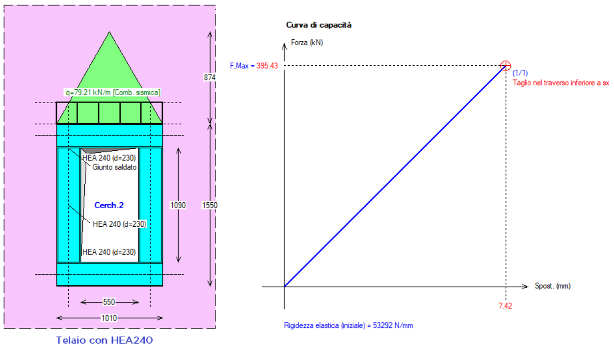
Fig. 17. Cerchiatura: telaio di rinforzo in acciaio con profilo HEA240 (PWF HEA240)
