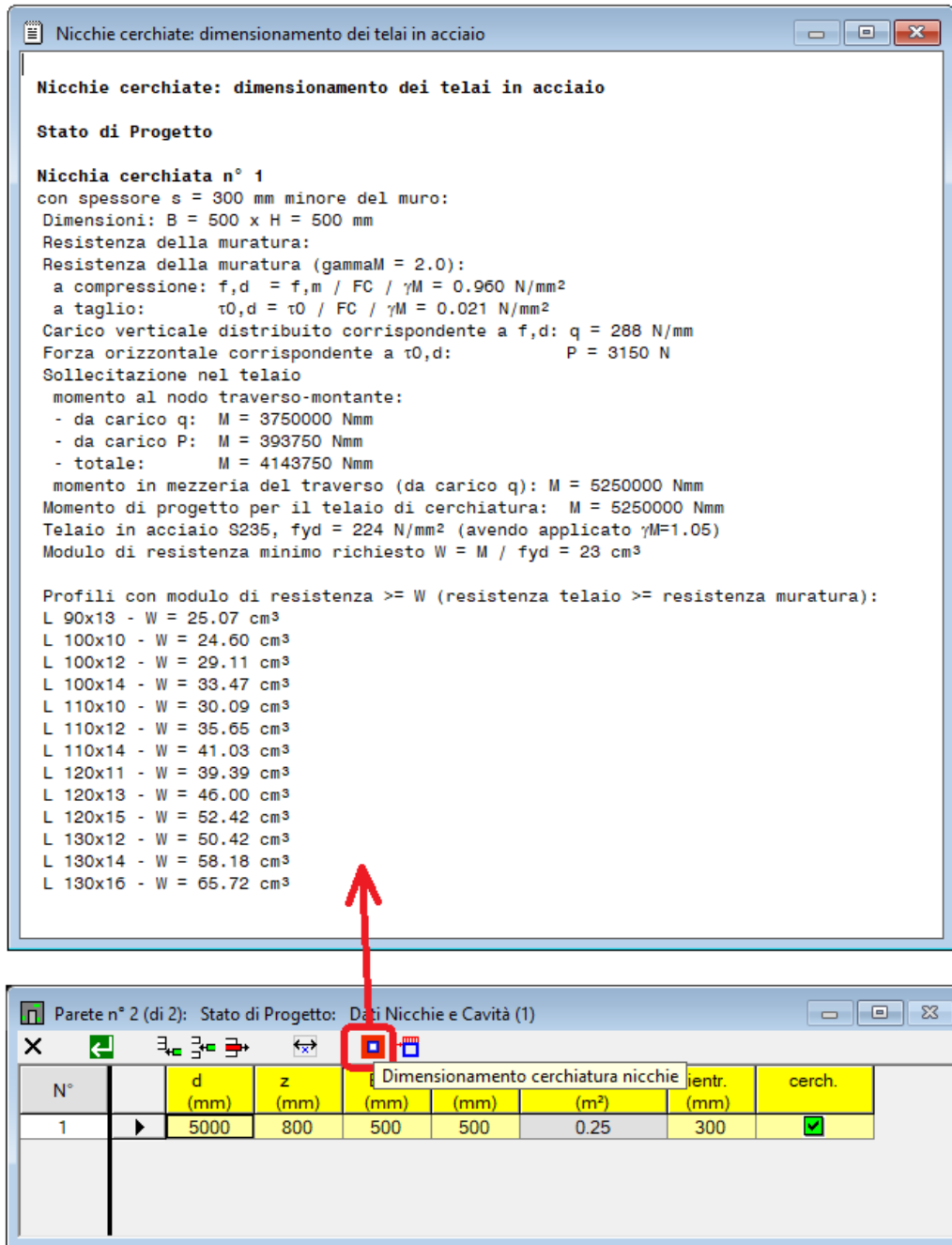
Fig. 9. Profili del telaio di rinforzo che compensano la perdita di resistenza dovuta alla nicchia
