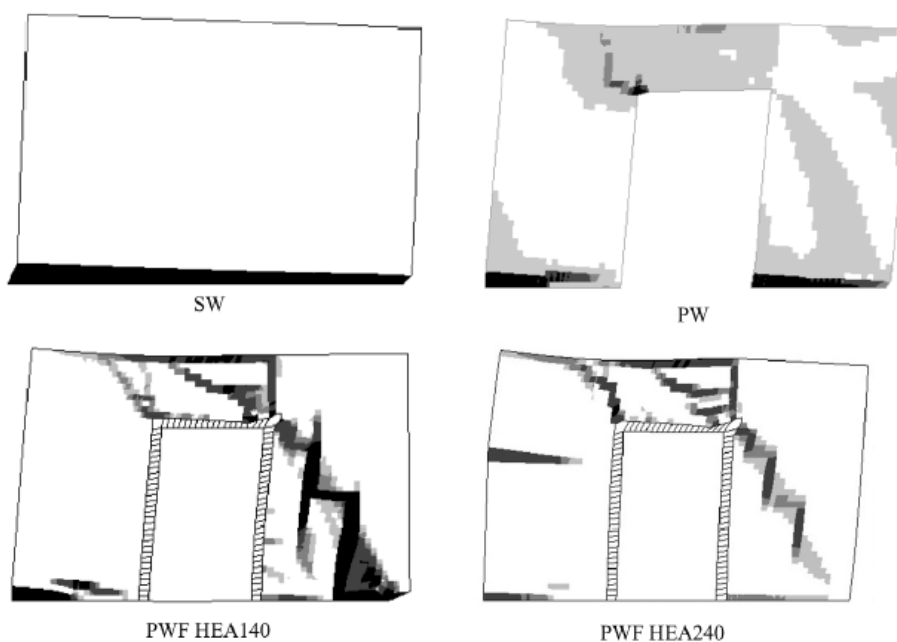
Fig. 8. Quadro fessurativo per i 4 casi esaminati (da [1])
