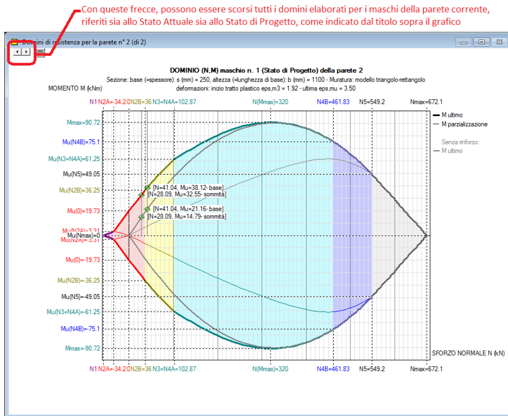
Fig. B.6.39. Dominio di resistenza per il maschio n°1 della parete di esempio rinforzato con FRCM
