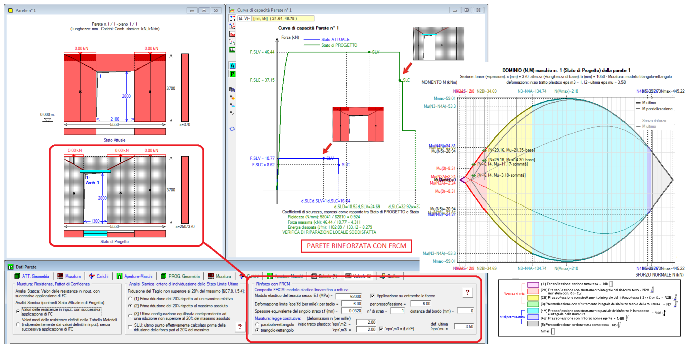
Fig. B.6.32. ACM: Intervento su singola parete per modifica apertura, con rinforzo in FRCM
