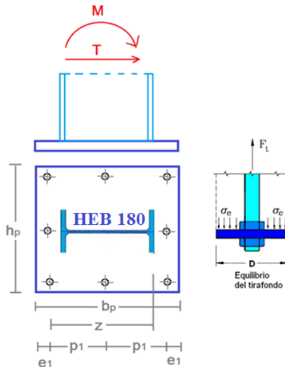
Fig. E.1.21. Geometria del giunto di base
