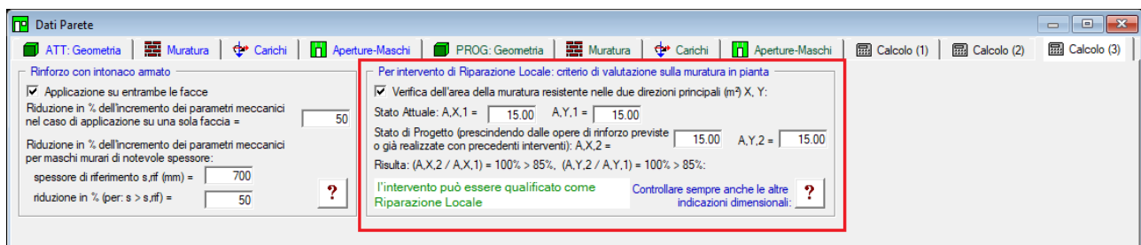
Fig. B.6.43. Criterio di valutazione sulla muratura in pianta per l'intervento locale
