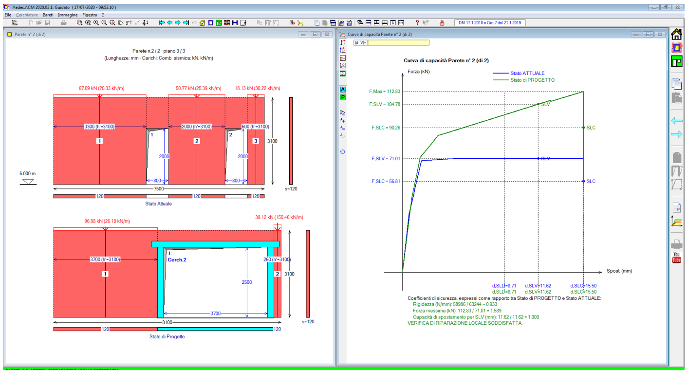
Fig. C.2.21. Verifica della parete n°2: Curva di capacità
