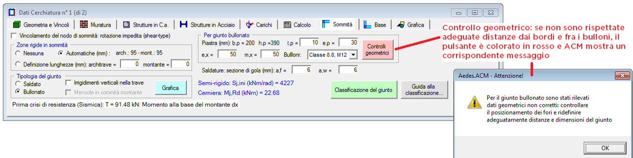
Fig. B.5.25. Finestra Cerchiature: scheda Sommità. Controlli geometrici sul giunto bullonato
