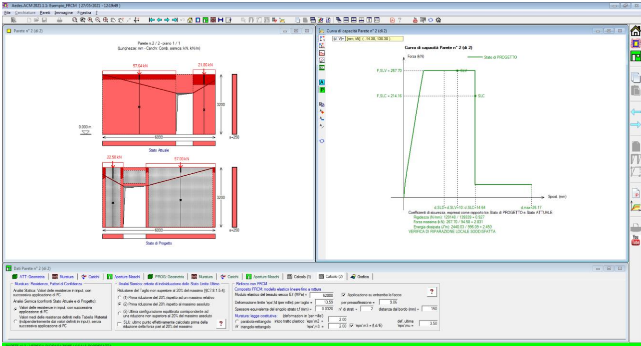
Fig. B.6.38. Risultati dell'analisi dell'esempio in caso di rinforzo con FRCM
