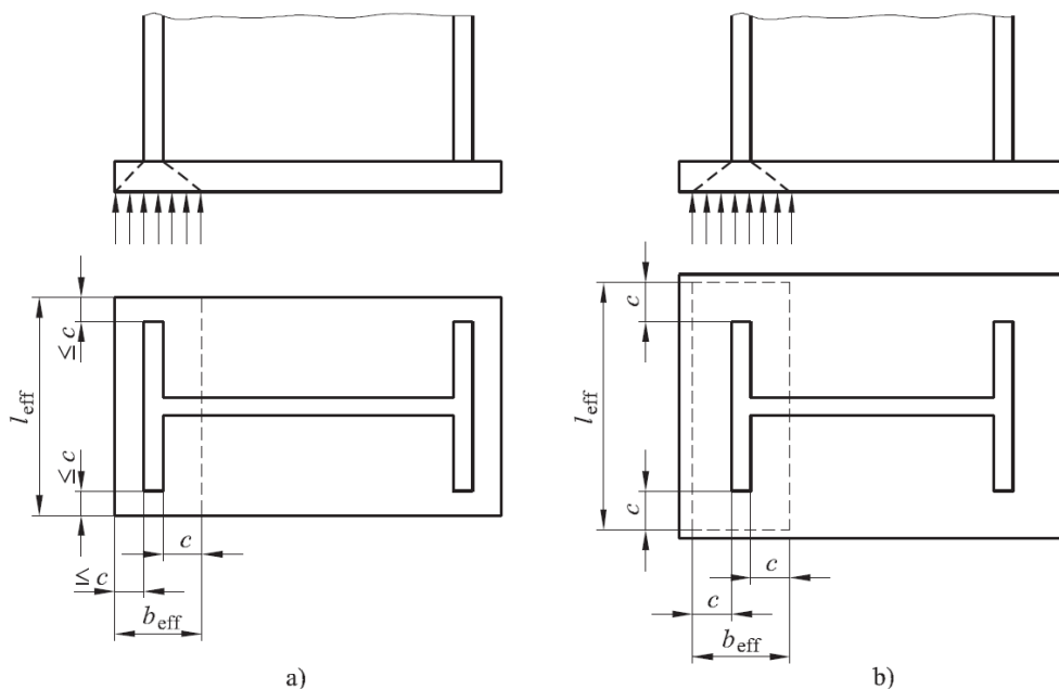
Fig. E.1.15. Area di un elemento T equivalente sollecitato a compressione
