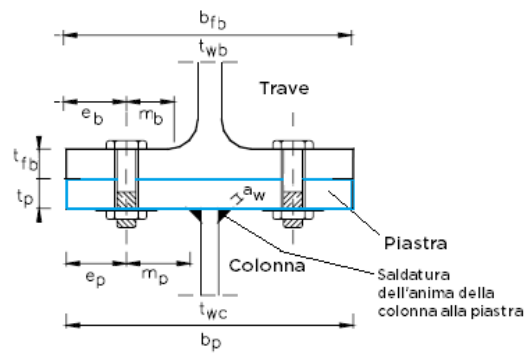
Sezione A-A
