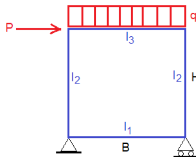
Fig. 3. Schema del telaio di rinforzo
