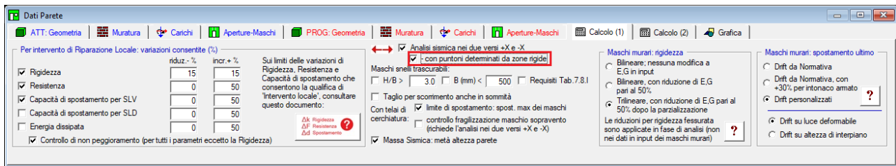
Fig. B.6.22. Analisi sismica nei due versi +X e -X: puntoni determinati da zone rigide
