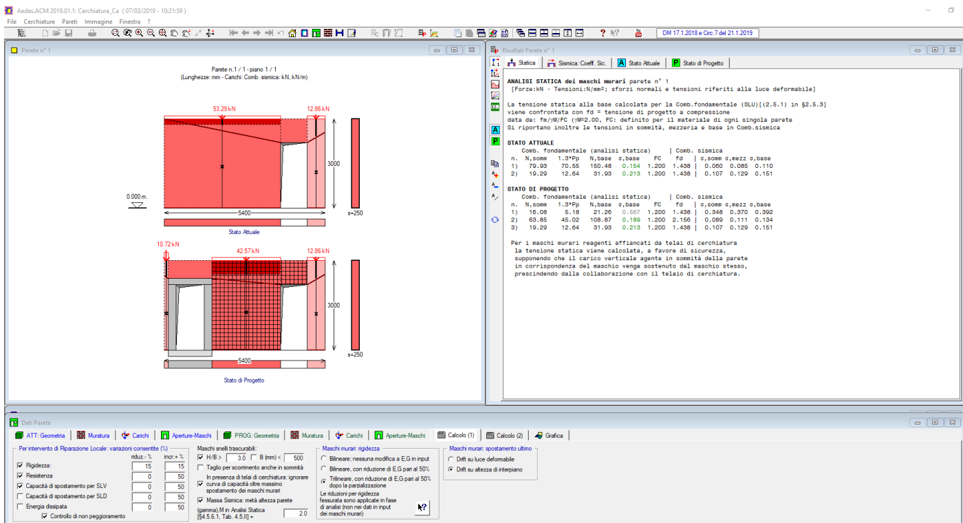
Fig. C.2.28. Parete contenente il telaio di cerchiatura in c.a.
