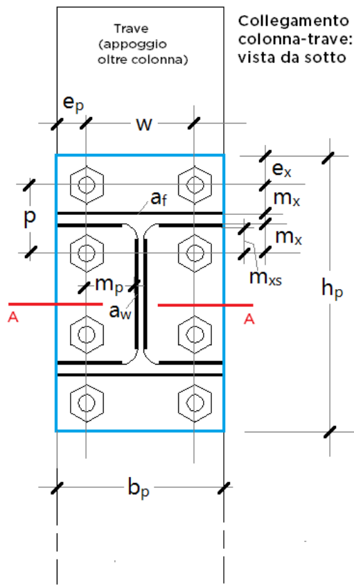
Fig. B.5.13. Giunto bullonato non irrigidito
