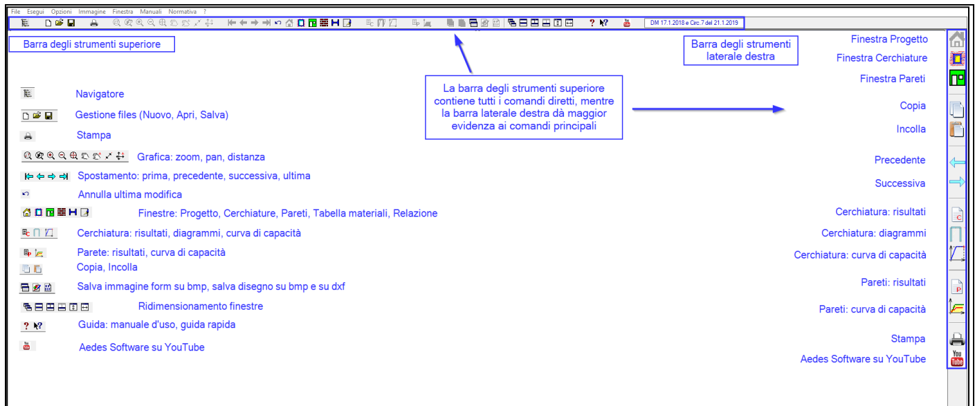
Fig. B.2.1. Barra degli strumenti: superiore e laterale destra
