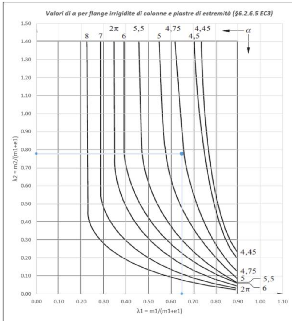
Fig. E.1.23 Determinazione del coefficiente \alpha
