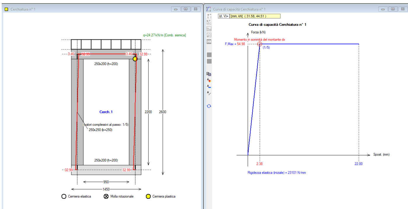
Fig. C.2.29. Curva di capacità del telaio
