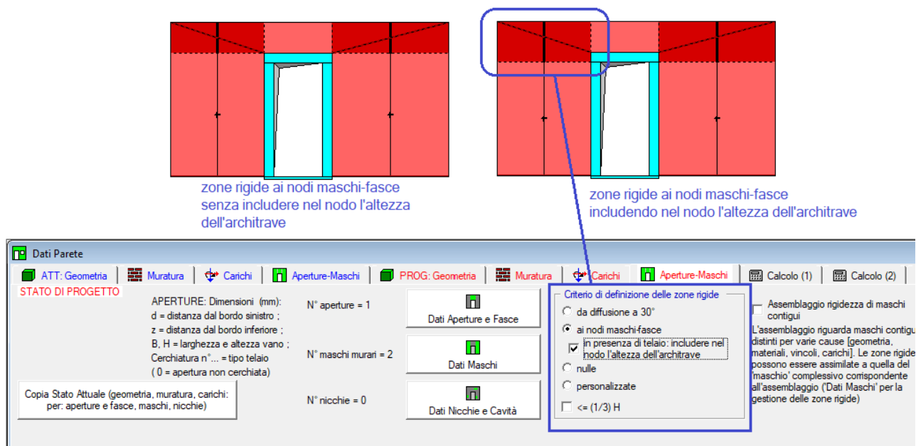
Fig. B.6.10. Zona rigida al nodo maschio-fascia: inclusione dell'altezza dell'architrave
