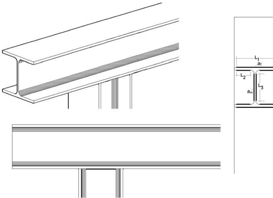
Fig. B.5.19. Giunto saldato non irrigidito
