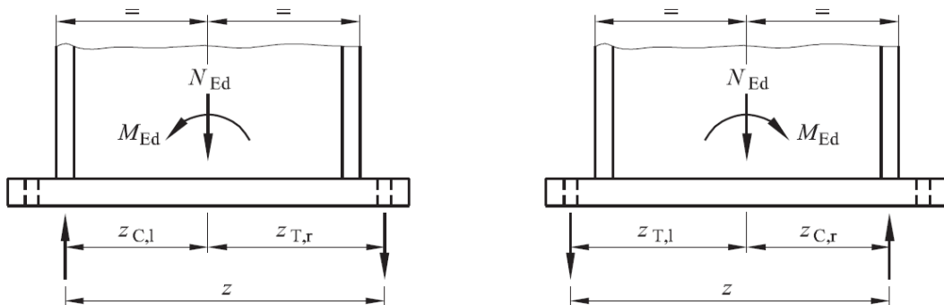
Fig. E.1.24. Area di un elemento T equivalente sollecitato a compressione
