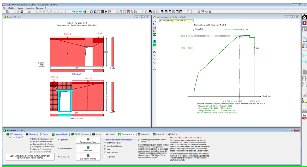
Fig. B.6.35. Esempio di studio per ACM: confronto fra cerchiatura e rinforzo con FRCM
