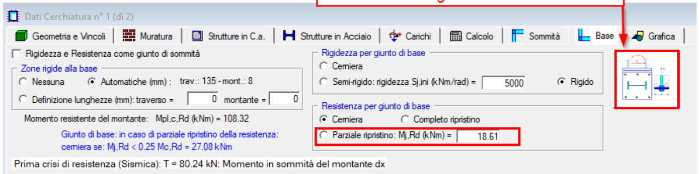
Fig. C.2.8. Giunto di Base.
