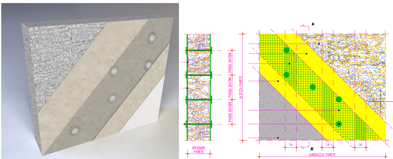
Fig. B.6.31. Rinforzo FRCM di un maschio murario
