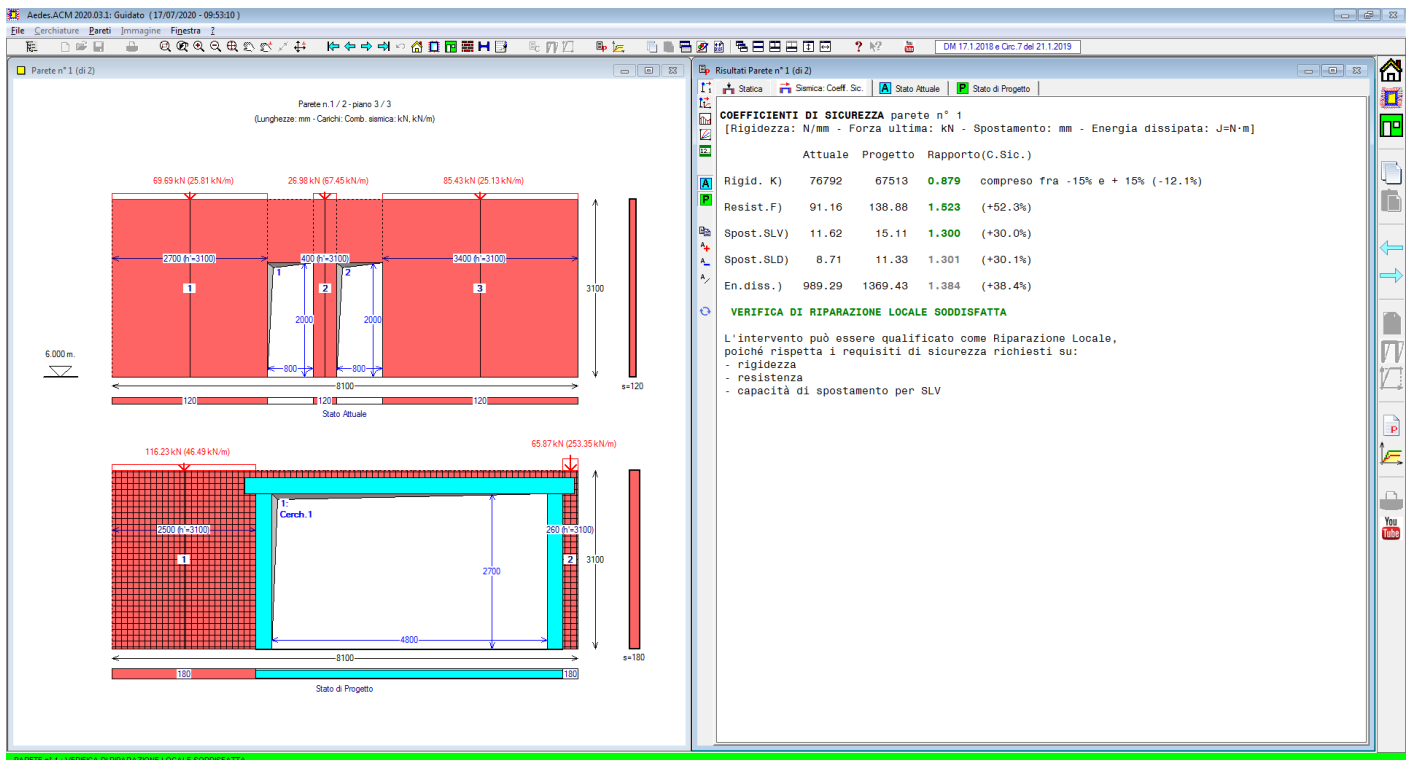
Fig. C.2.17. Risultati Parete n°1
