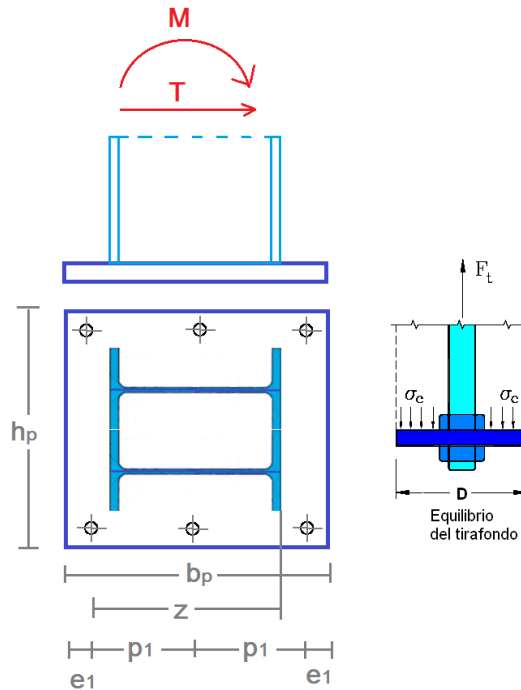
Fig. E.1.7. Giunto di base
